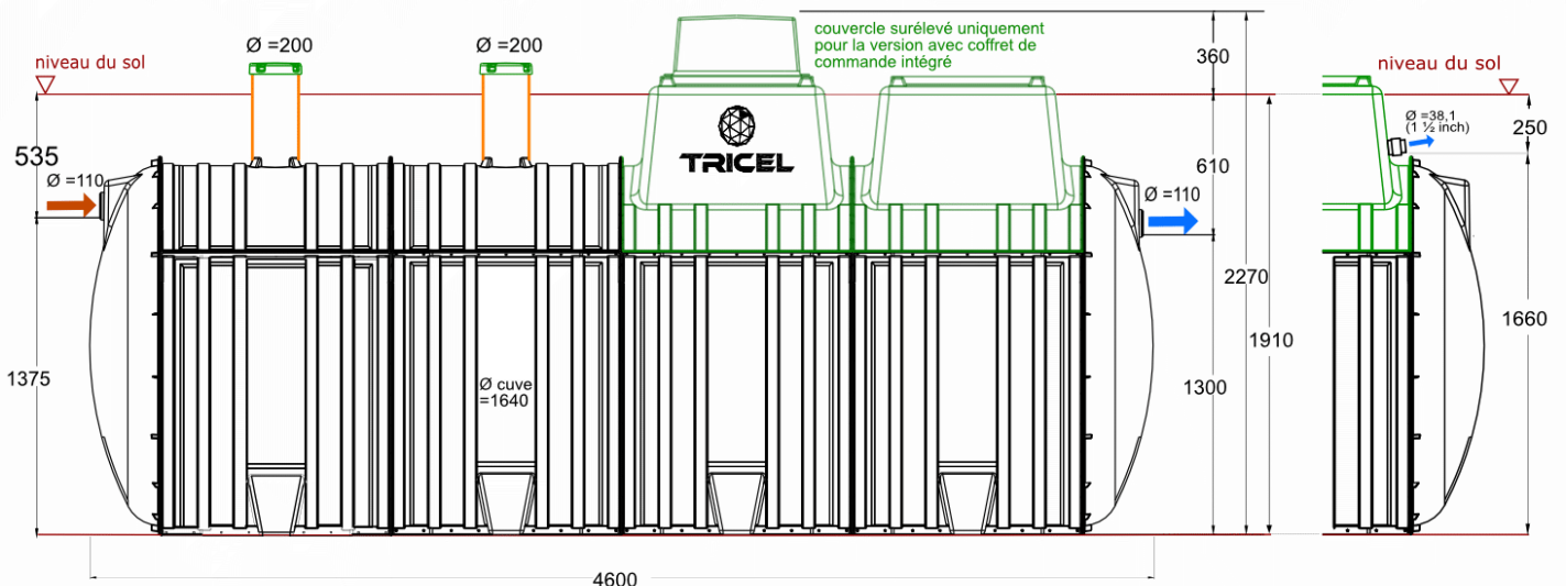
Tricel Novo 10 EH avec écoulement gravitaire (naturel)
