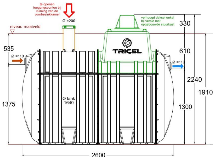
Tricel Novo 6 IE met gravitaire (natuurlijke) afvoer
